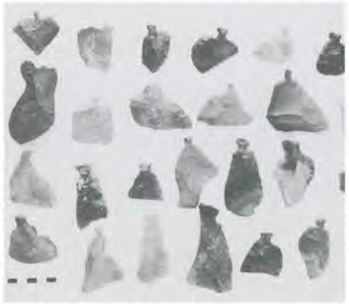
▲小館遺跡から発掘した石器
