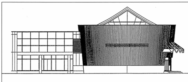
南西側立面図
