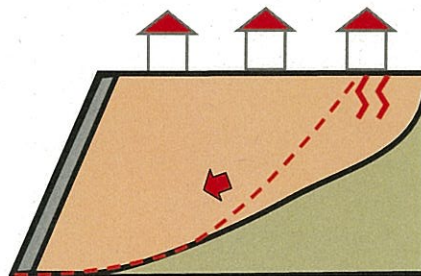
図 I.3 腹付け型大規模盛土造成地で発生する滑動崩落のイメージ
