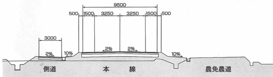
標準断面図
